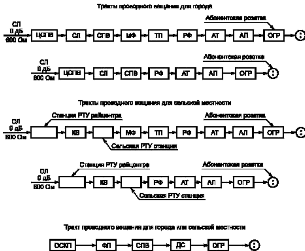
Рисунок А.1 — Структуры трактов проводного вещания
