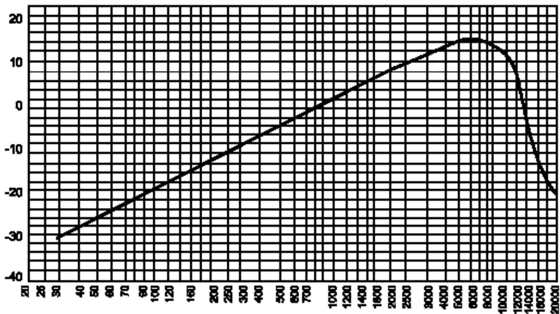
Рисунок 19 — График АЧХ псифометрического фильтра в соответствии с [1]
